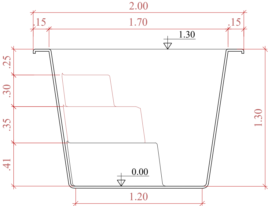
CORTE TRANSVERSAL SEM ESCALA
