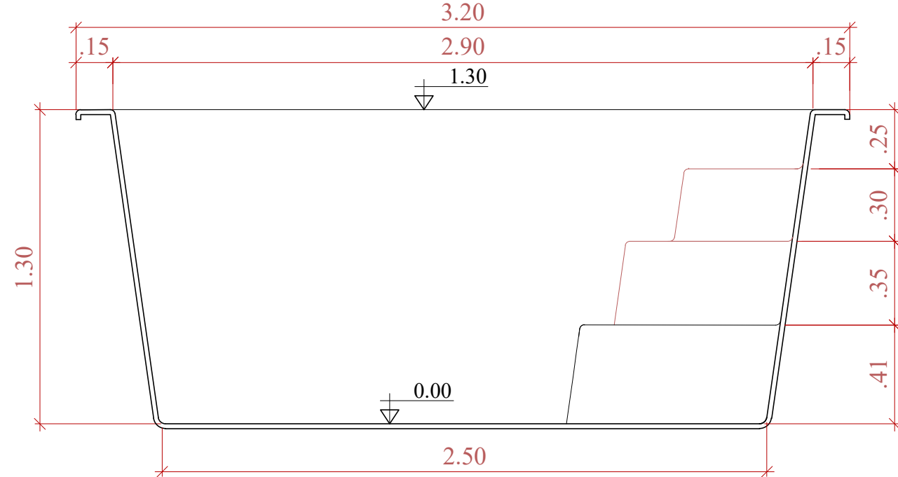
CORTE LONGITUDINAL SEM ESCALA
